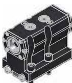
Doppel-Aufnahmehalter double tool holder
