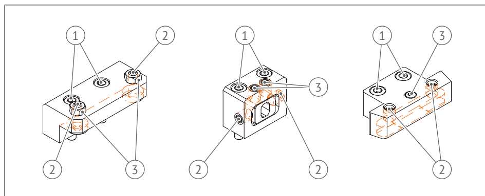
Abb. 19: Voreinstellbare Fixierung
