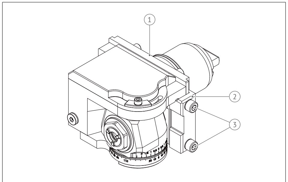
Abb. 15: Befestigungsmittel Keilleiste
