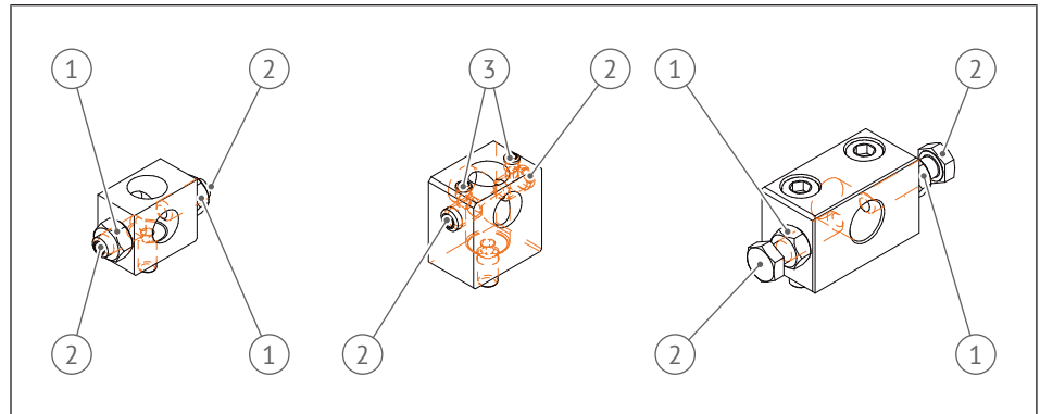
Abb. 18: Einstellbare Fixierung
