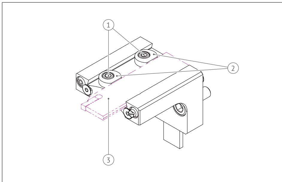
Abb. 33: Klemmscheibe
