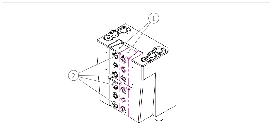
Abb. 30: Drehstahlhalter: Doppelte Nut
