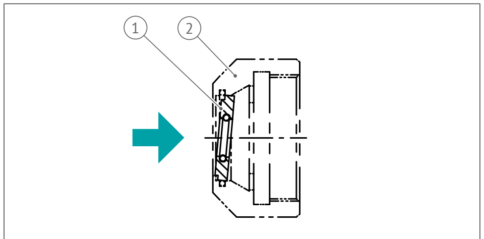
Abb. 22: Ausführung DS/ER: Dichtscheibe demontieren
