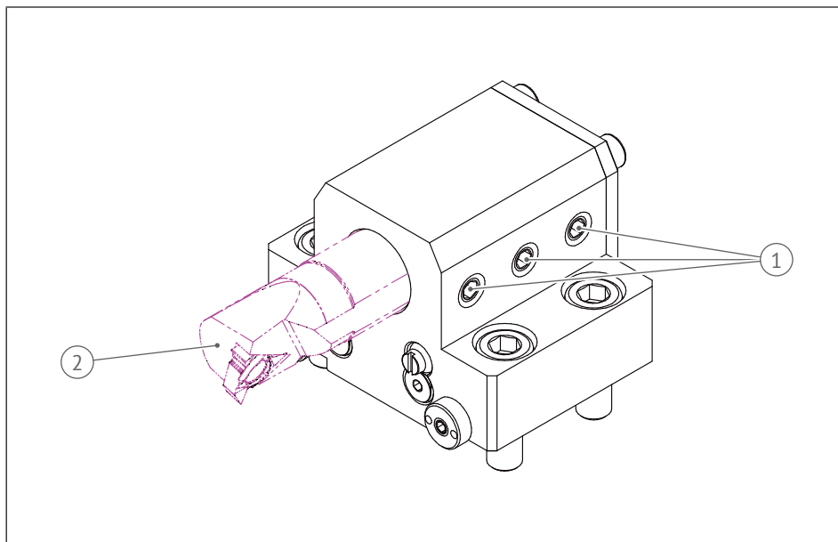
Abb. 31: Gewindestifte
