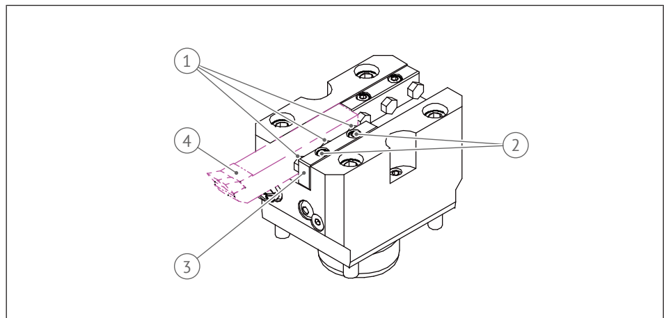
Abb. 29: Leiste mit Sechskantschrauben
