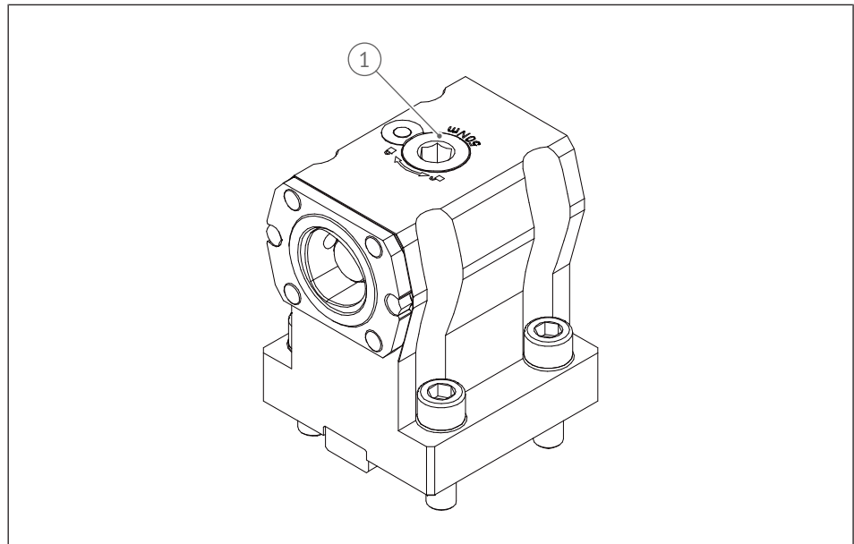
Abb. 25: heimatec.Capto™ Werkzeughalter
