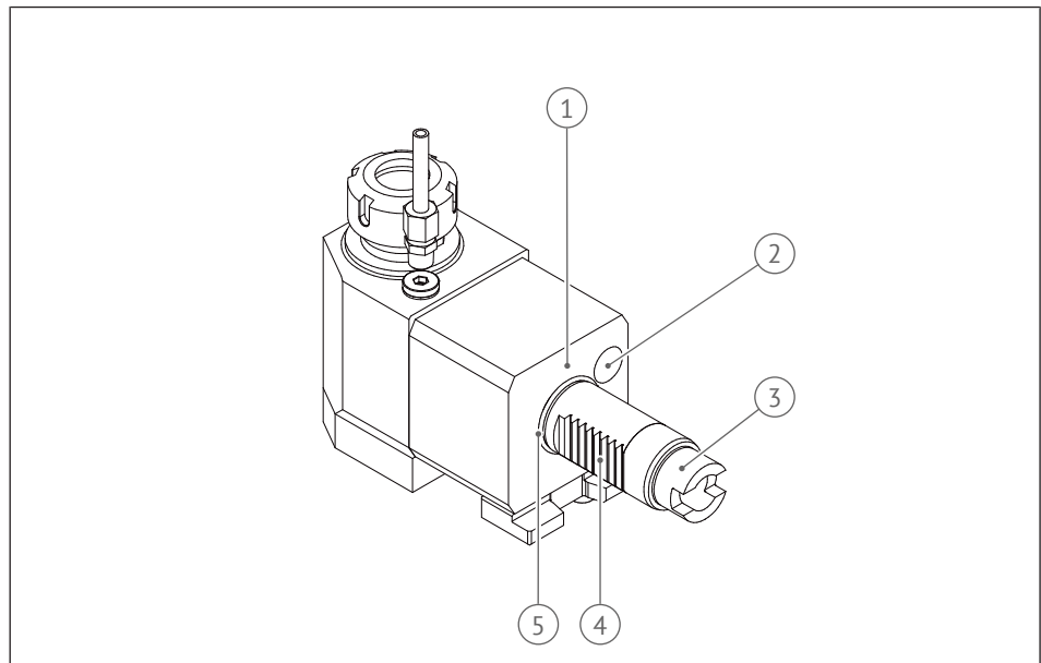
Abb. 6: VDI-Schnittstelle
