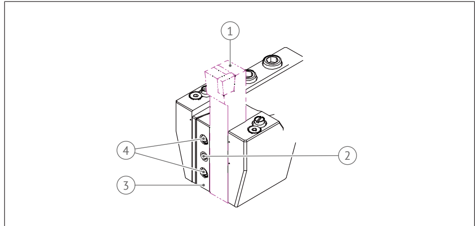
Abb. 28: Keilleiste
