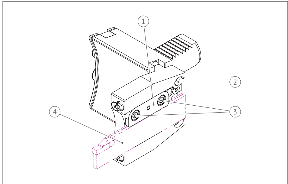
Abb. 35: Höhenverstellung
