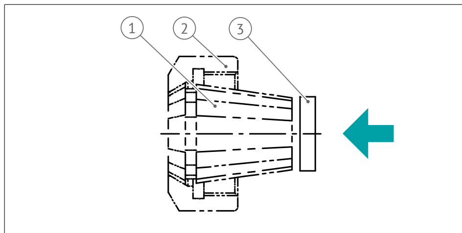
Abb. 23: Ausführung heimatec-DS
