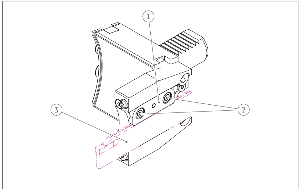
Abb. 34: Klemmleiste
