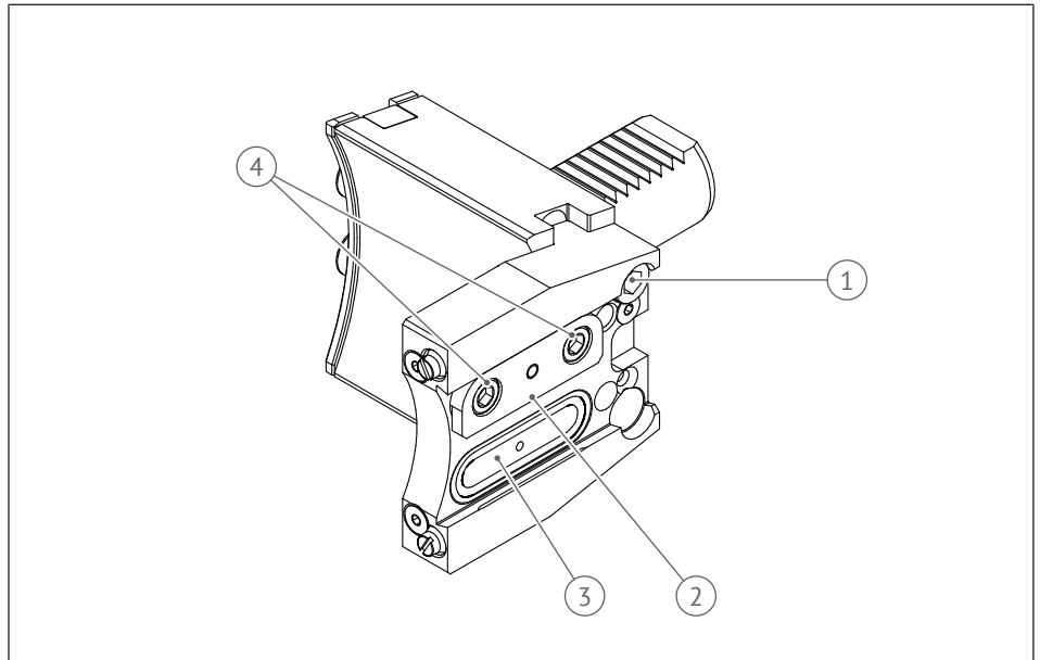
Abb. 36: Abstechhalter: Doppelte Nut
