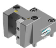
Kombi-Drehstahlhalter (8 224 15 006)
