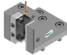
Drehstahlhalter (8 224 15 002)
